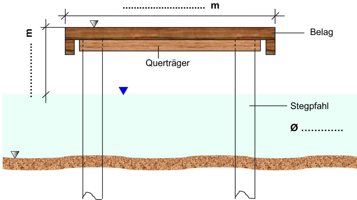
Querschnitt
